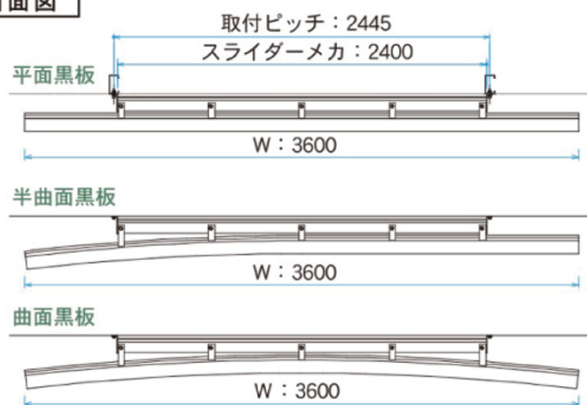
横断面図
