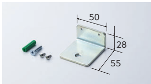
●YKU-1の使用例
