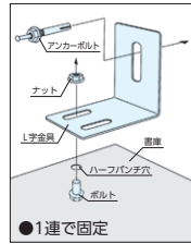
●TKU-2 1連での使用例
