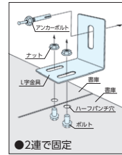
TKU-1又はTKU-2の使用時に天面にハーフパンチ穴をあける場合は所定の位置にドライバーを充てがいハンマーでたたき、穴をあけてください。
