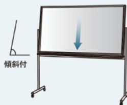
MV36TMN ¥53,600 外形寸法/W1902×D610×H1810 板面寸法/W1810×H910 有効寸法/W1770×H870
