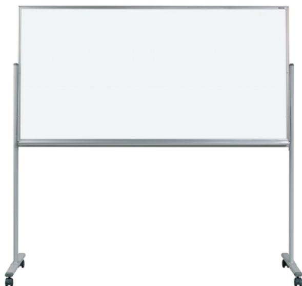
MV36TN ¥49,600 外形寸法/W1902×D610×H1810 板面寸法/W1810×H910 有効寸法/W1770×H870
