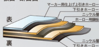
板面 断面図
