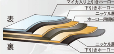
板面 断面図
