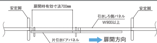
片引きドア取付例 (右引き扉)
